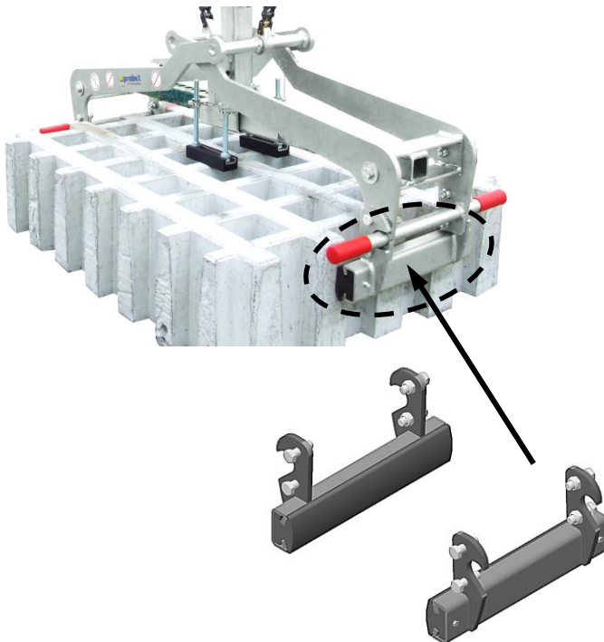
FTZ-MULTI-15 mit Greifbacken WB-SQ (für Steinquader) (43100941)
