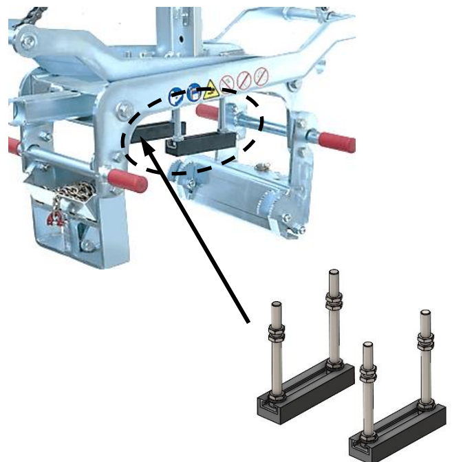
Höhenverstellbare Auflage HVA-FTZ/TSZ (43100867)
