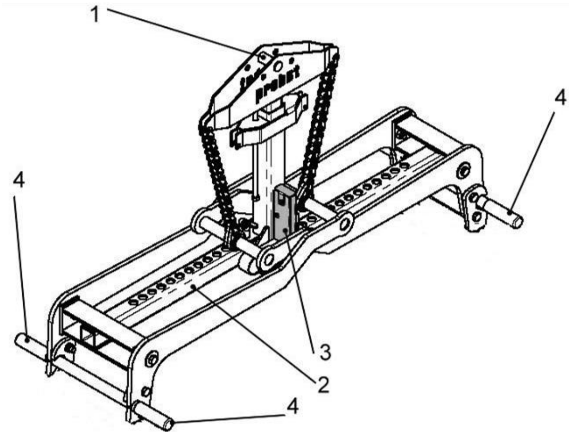
Fig.1 (Unidad básica FTZ-MULTI-15/sin mordazas)
