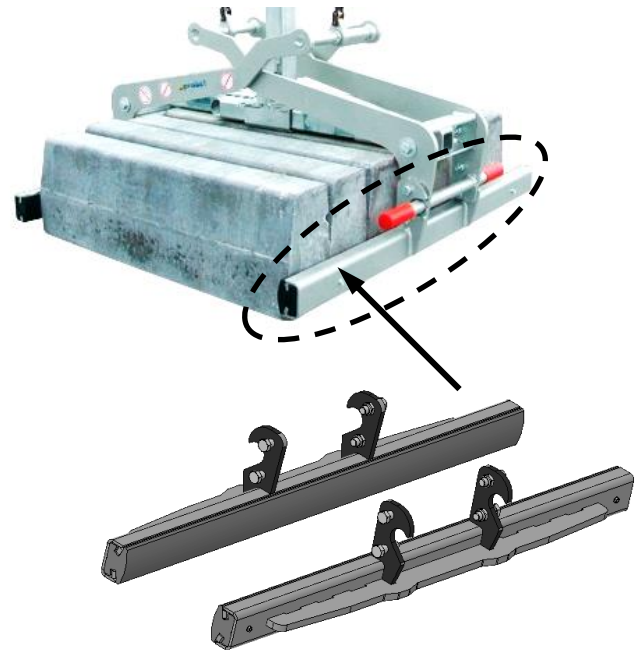
FTZ-MULTI-15 mit Greifbacken WB-G-120 (43100943)
