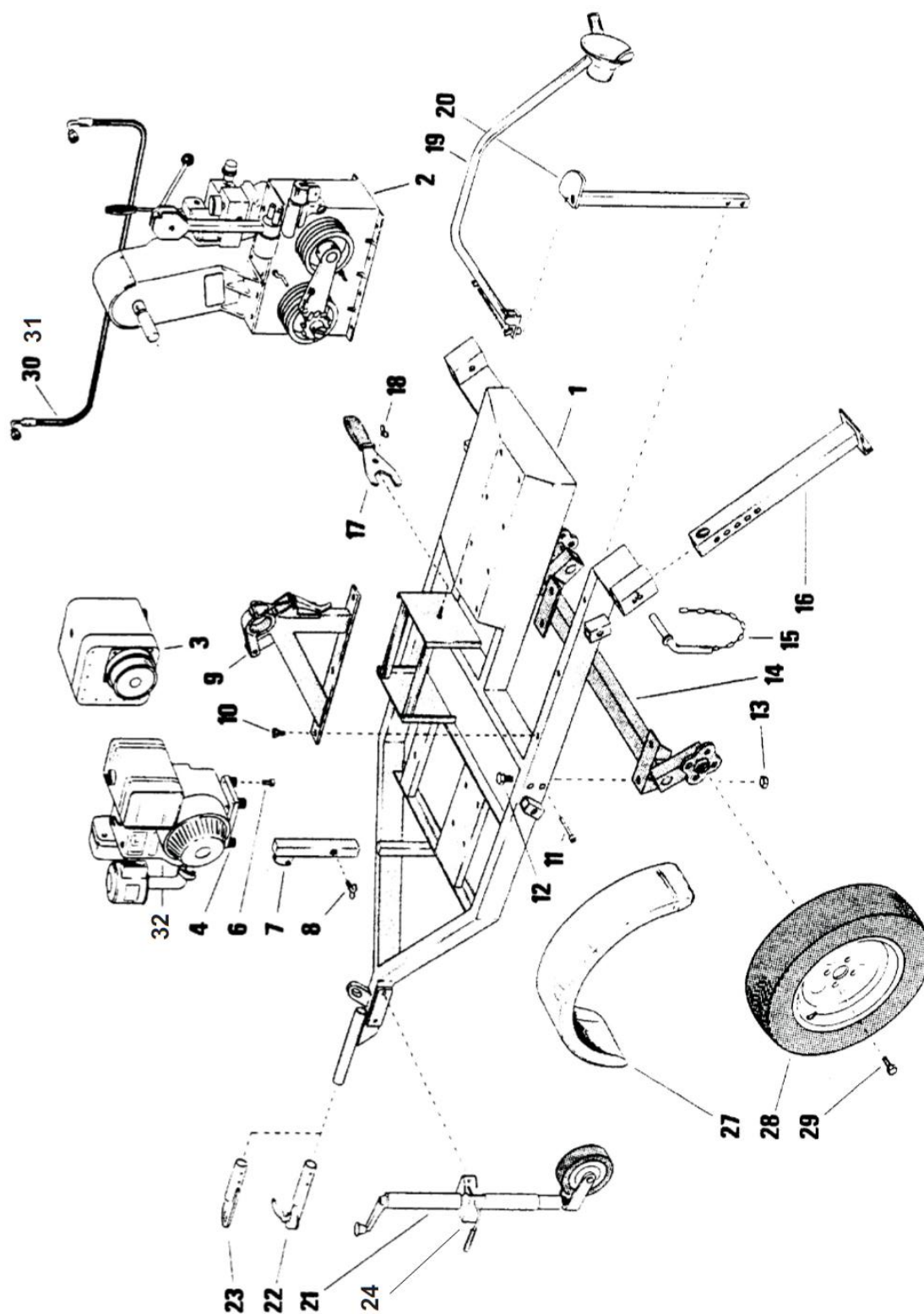
Sprängskiss chassi
