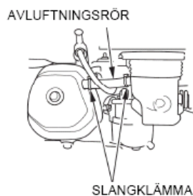
MODELL MED FÖRGASARE MED INTERN VENTIL
