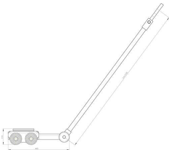
JLB 6 K | Bestell-Nr. 07 061 085-V | Seitenansicht JLB 6 K | Order No. 07 061 085-V | Side view
